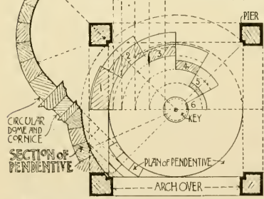
BYZANTINE & RENAISSANCE DOMES
