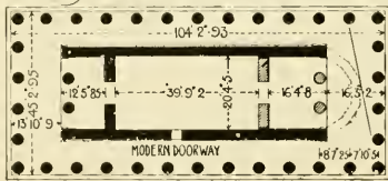
(D) PLAN
