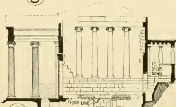
(D) SECTION XXIX (AFTER MIDDLETON, UNRESTORED)
