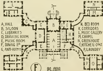
(F) PLAN
