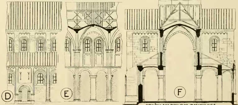
PART EXTERIOR ELEVATION (D)
